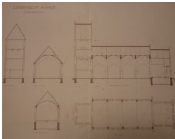
Tegning dateret 1931, visende snit og fundament af den oprindeligt tænkte kirke uden krypt. Tegning opbevares hos Sundby-Samlingerne.
